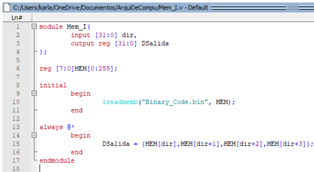
Módulo Mem_I en ModelSim.
